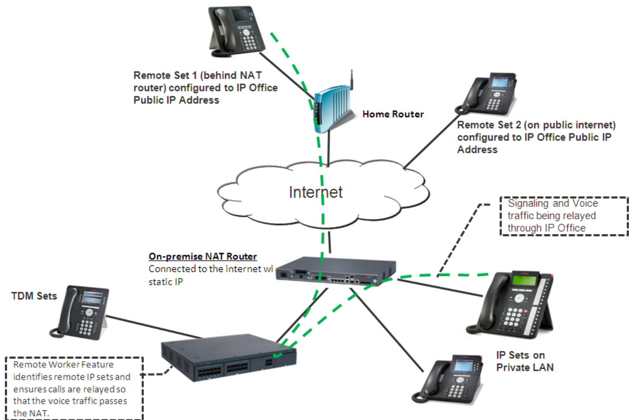
Abbildung 1: Remote Worker-Interaktionen
